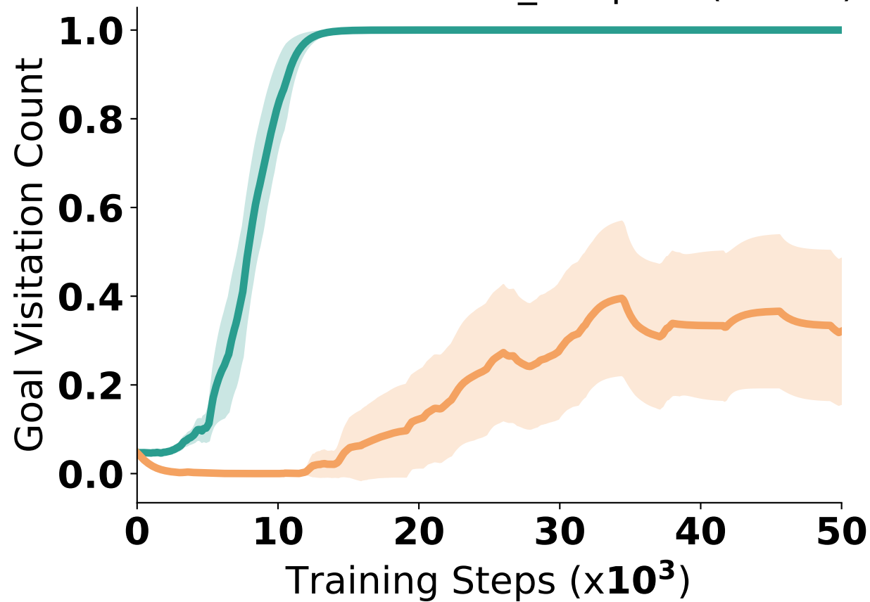
Gridworld-Bottleneck_NExperts(20.0%)
